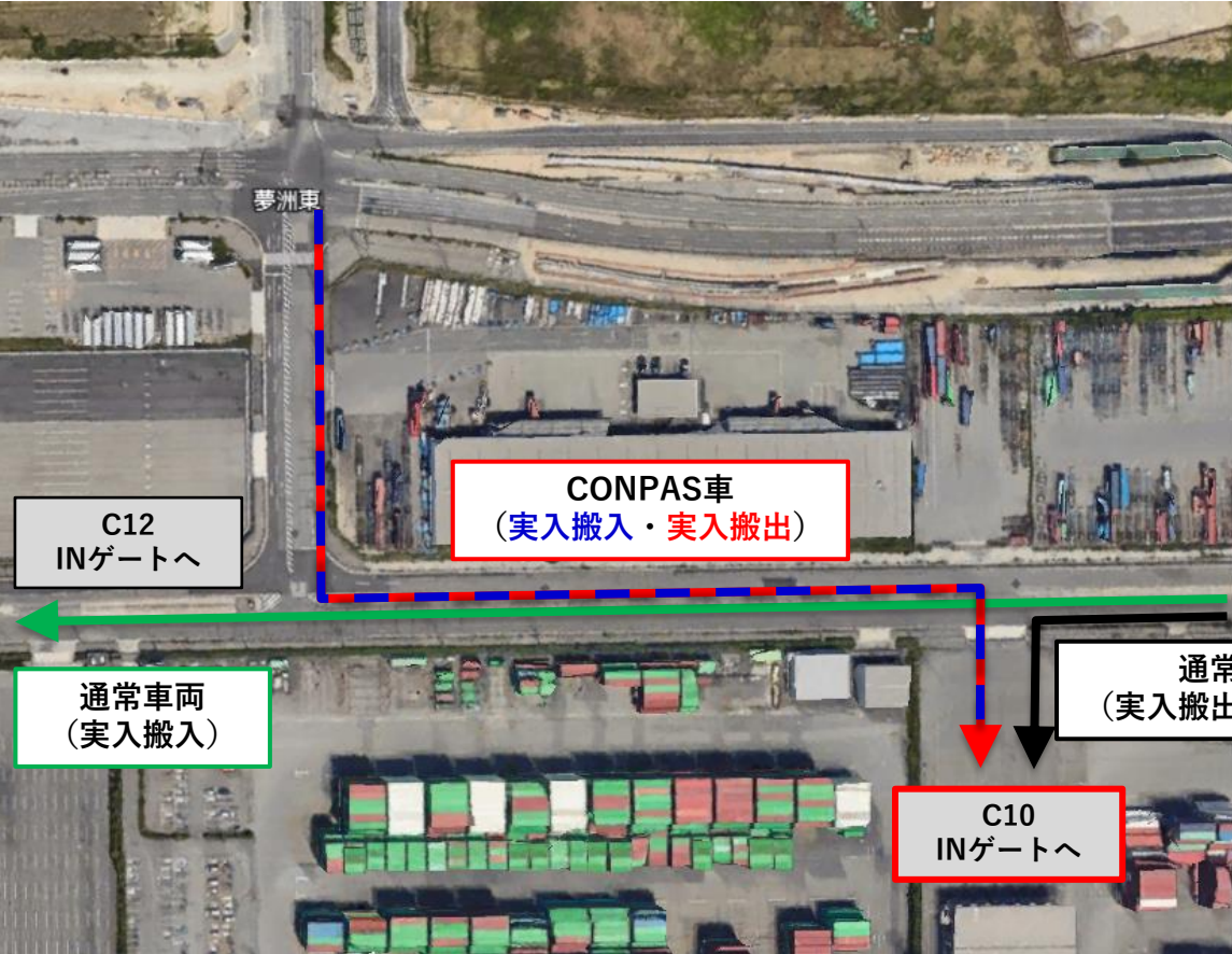
CONPAS車動線
